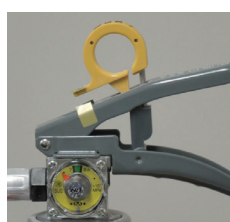
× 安全栓の抜けかけ
