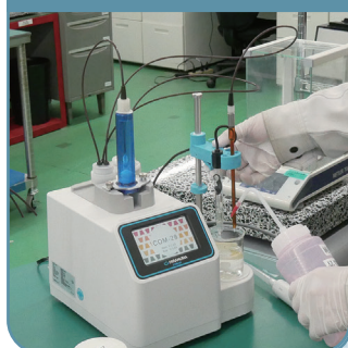
自動滴定装置 COM-28
