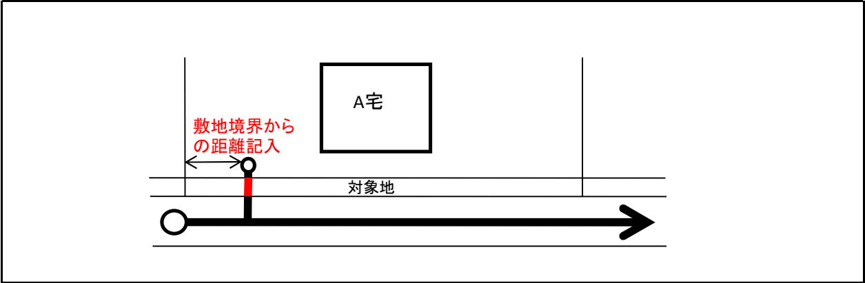
公共ます設置位置図
