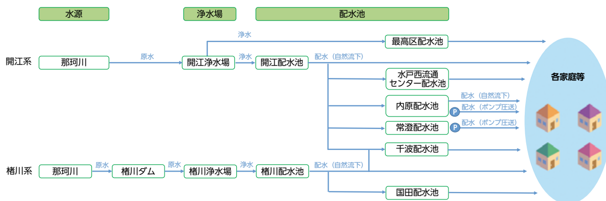
図2-1-2 主要な水道施設の系統フロー
