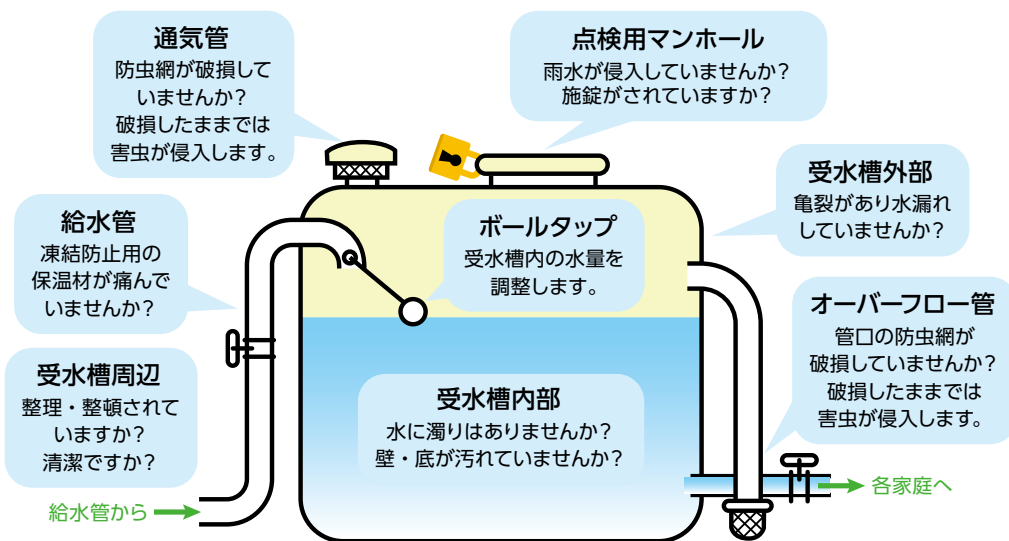
図4-1-9 貯水槽水道の管理のポイント
