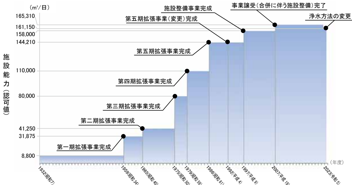
図2-1-1 施設能力(認可値)の推移
