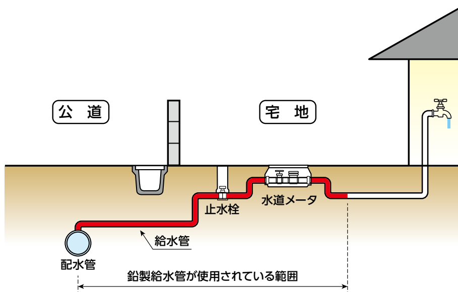
図4-1-4 鉛製給水管解消範囲図（例）
