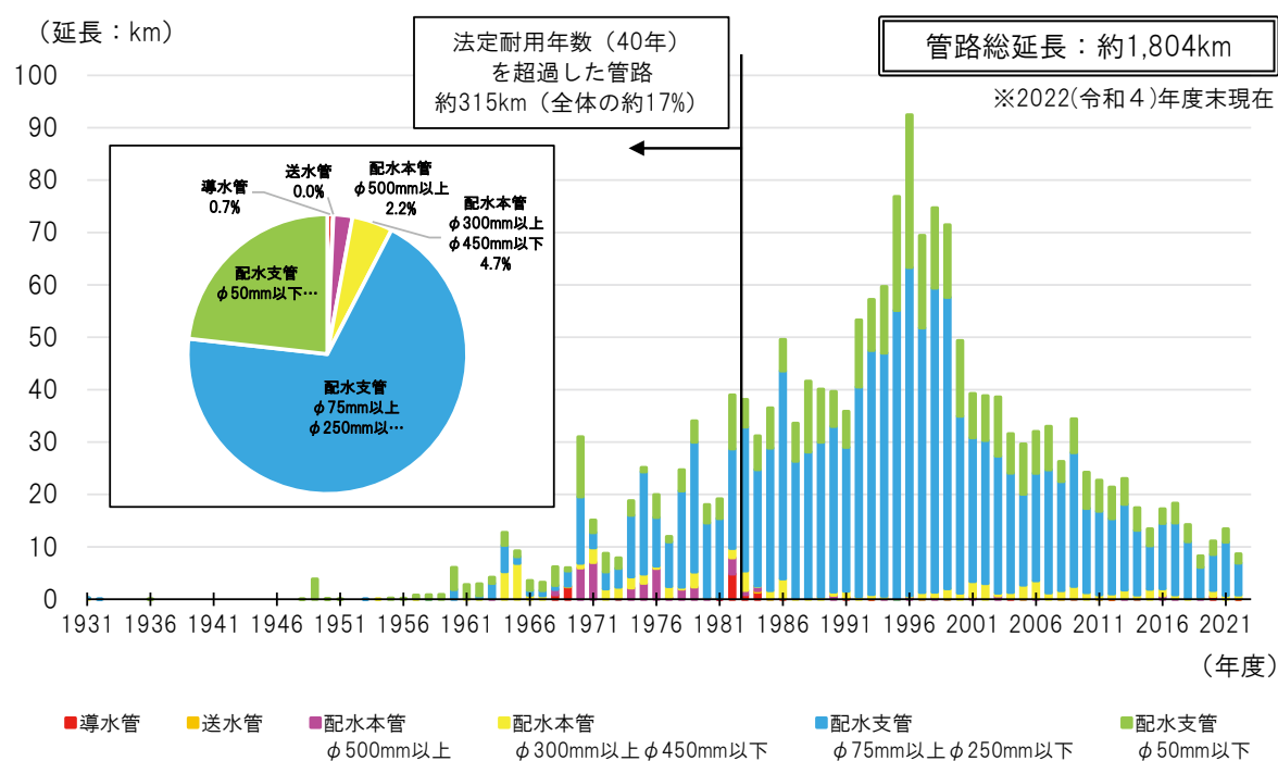
図4-2-2 年度別・用途別管路延長
