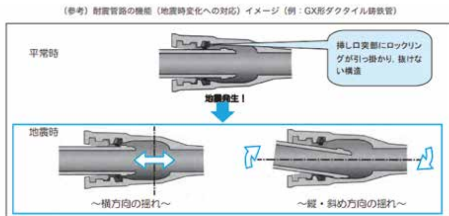
図4-2-6 耐震管路の構造
