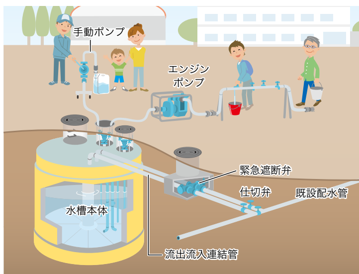
図4-3-2 耐震型循環式飲料水貯水槽のイメージ
