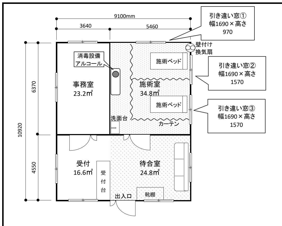
施術所平面図(例)
