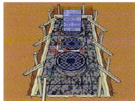
⑭上部スラブコンクリート 型枠、配筋 鉄筋 D=〇〇, ㊦=〇〇
