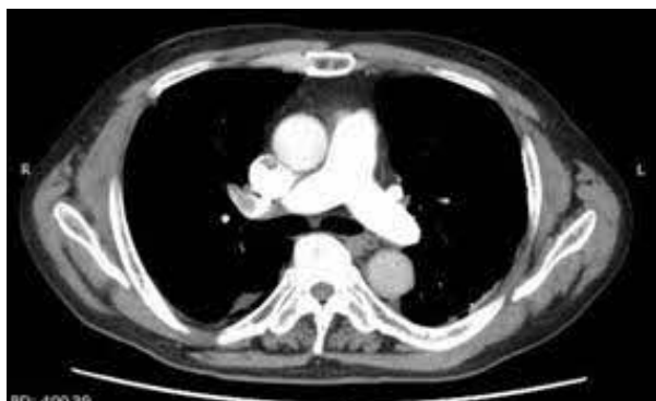
造影 CT
