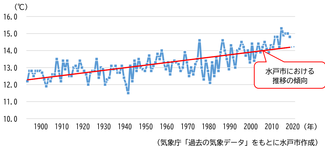
〔図4-10〕 水戸市の年平均気温の推移
