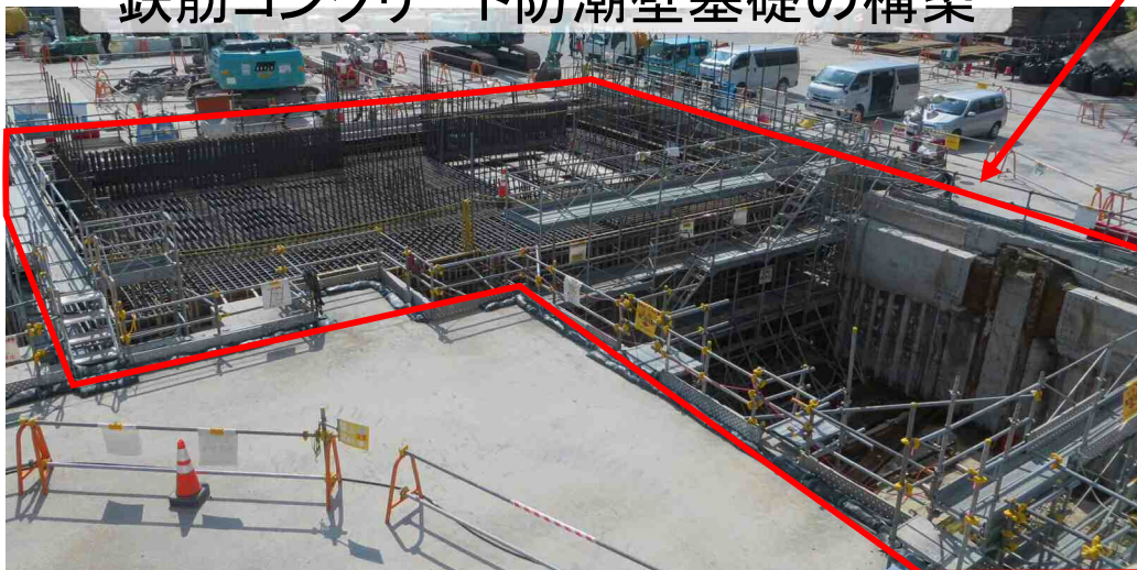
鉄筋コンクリート防潮壁基礎の構築
