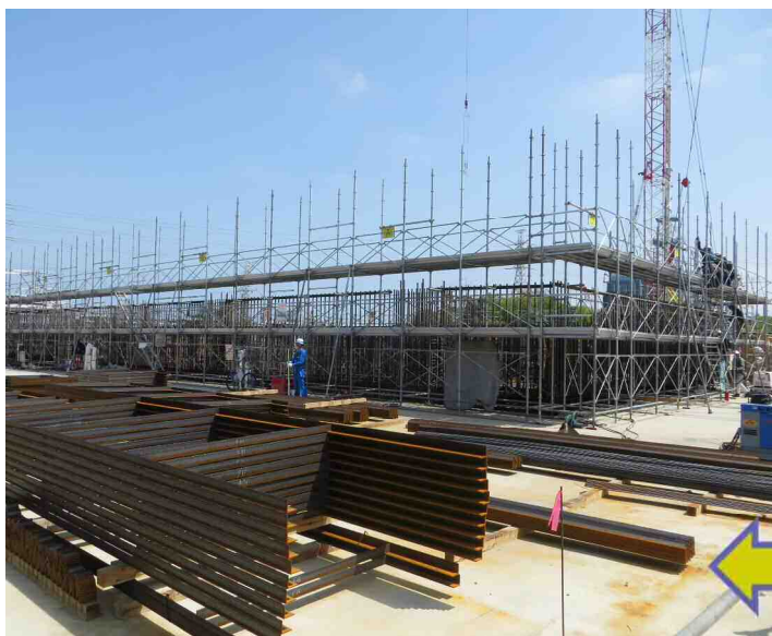
緊急時対策所建屋 建屋構築
