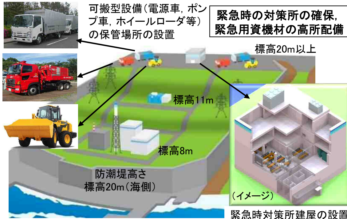
高台の整地時
