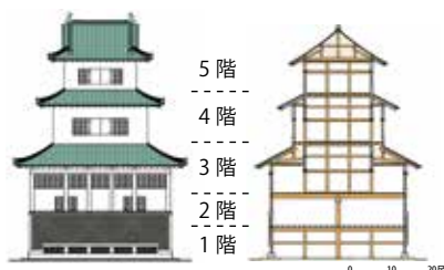
◀三階櫓立面図(左)・内部構造図(右)
