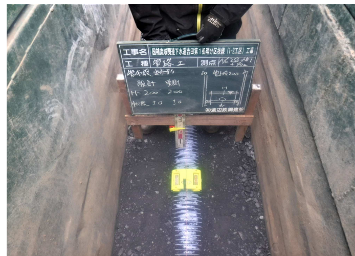
No.30 (有)渡辺鉄鋼建設 国補流域関連下水道吉田第1処理分区枝線(1-2工区)工事
