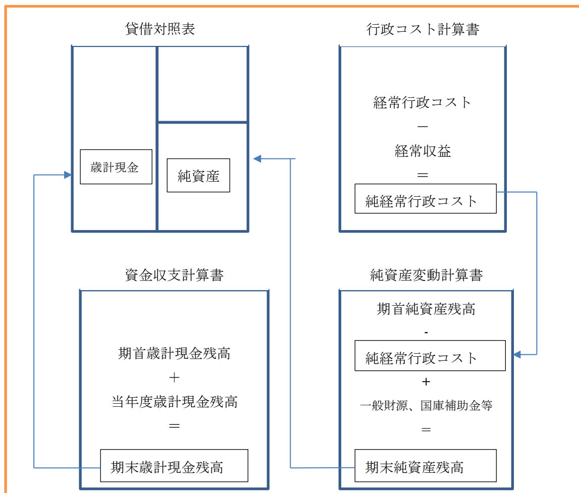
4 表の相関図
