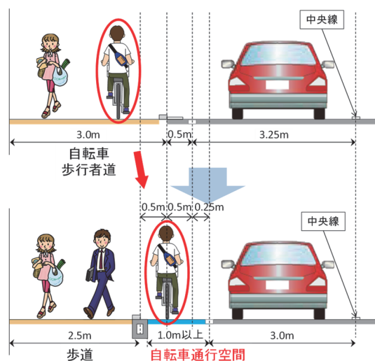
図 4-7 自転車歩行者道の見直しイメージ
