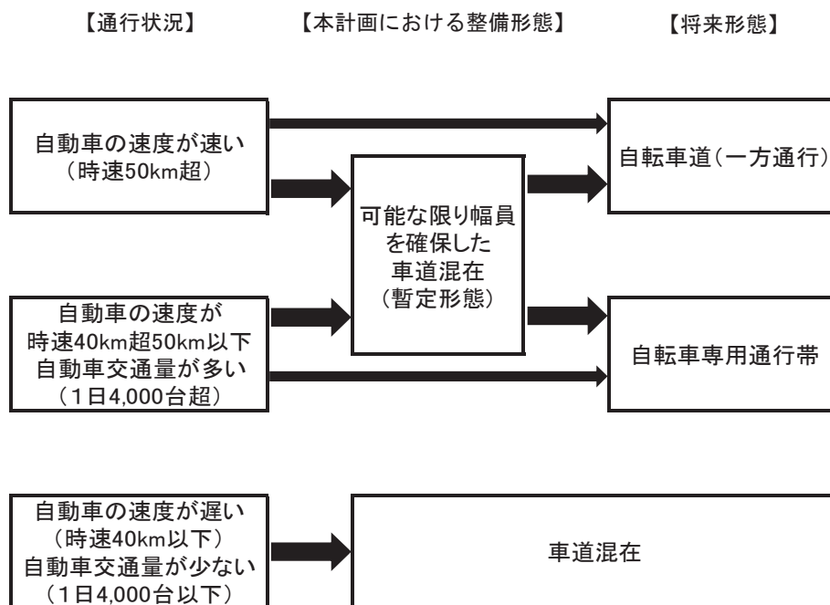
図 4-4 整備形態の選定の考え方
