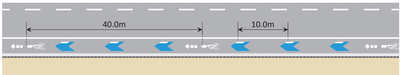
図 4-9 一般単路部における路面表示方法
