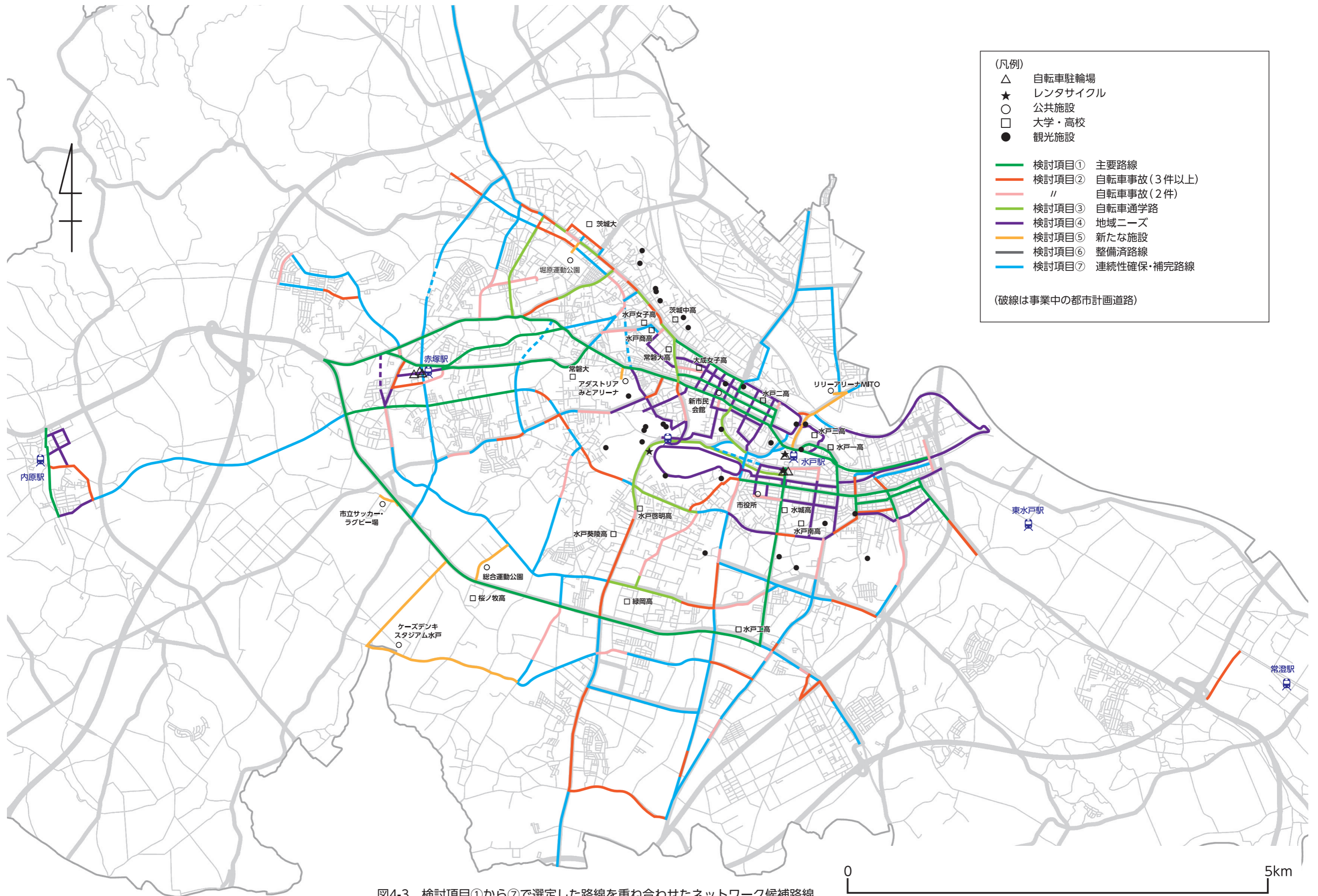
図4-3 検討項目①から⑦で選定した路線を重ね合わせたネットワーク候補路線
