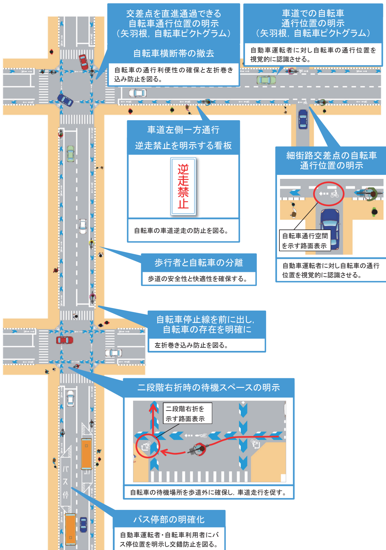
図 4-21 整備後のイメージ
