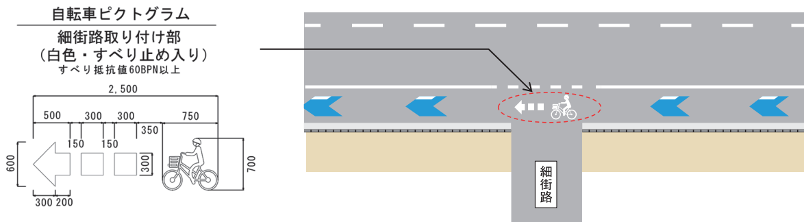
図 4-11 細街路との交差点における路面表示方法
