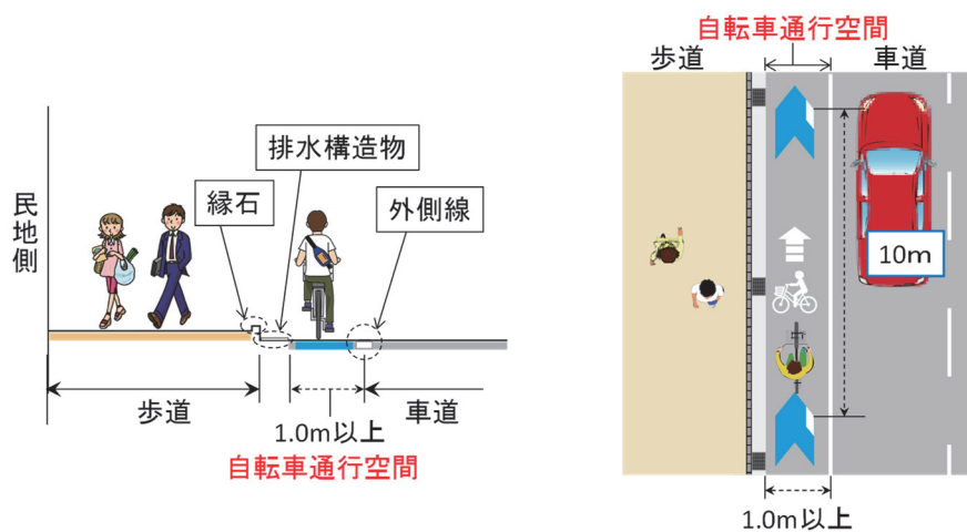
図 4-17 路肩幅員を十分に確保できる場合(車道混在の標準形)の整備方針
