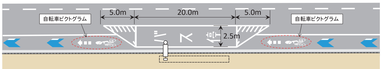
図 4-12 バス停留所付近における路面表示方法
