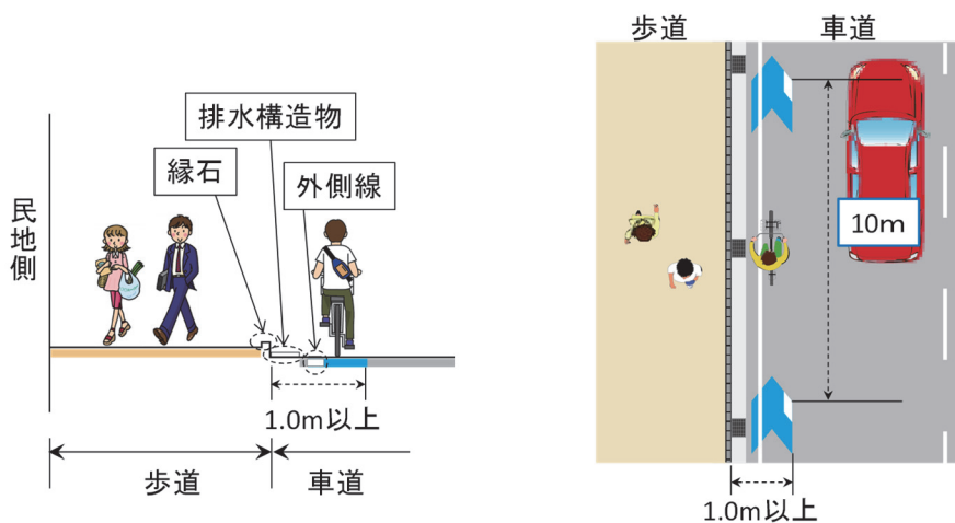
図 4-18 路肩幅員を十分に確保できない場合の整備方針
