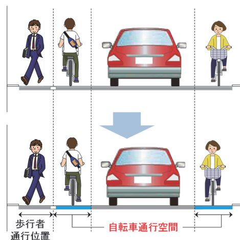
図 4-6 狭い道路の整備イメージ
