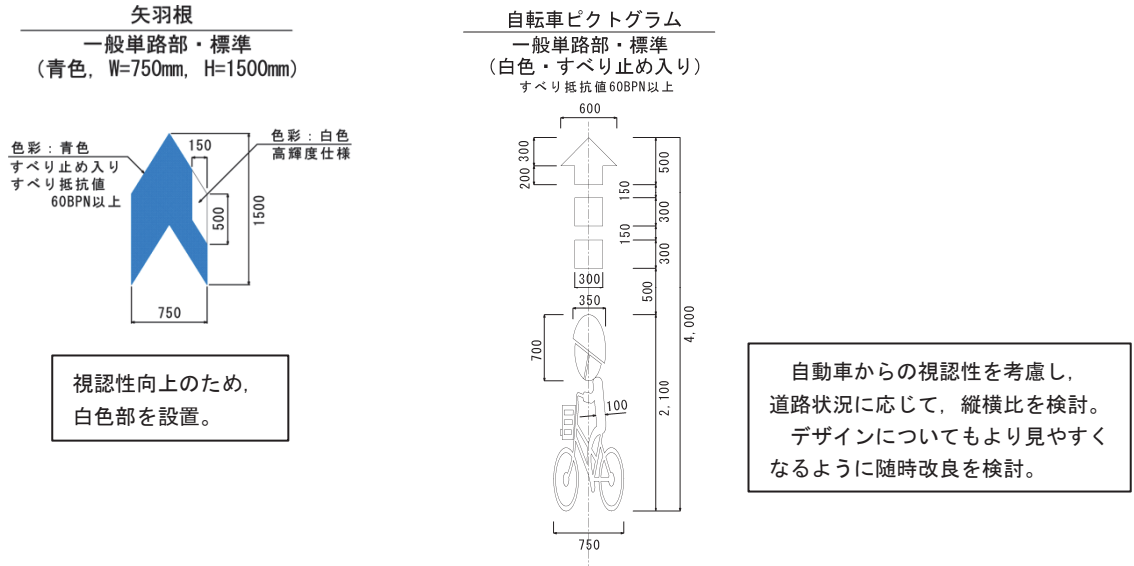
図 4-8 ネットワーク路線で使用する主な路面表示
