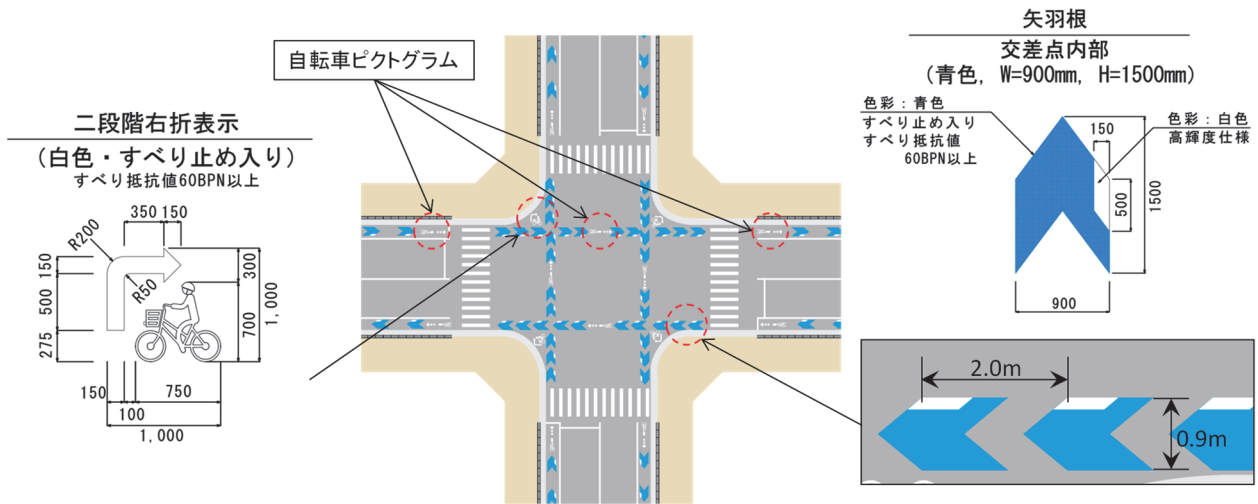
図 4-10 交差点における路面表示方法
