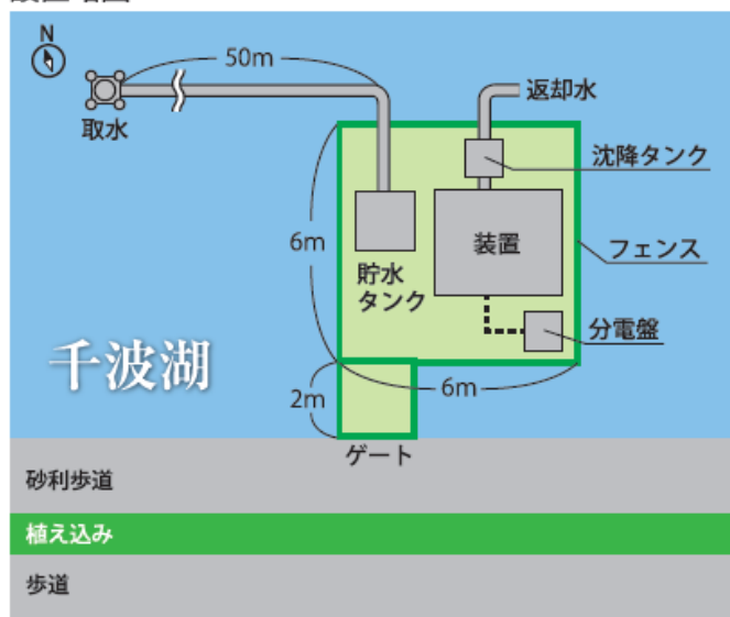
設置略図
