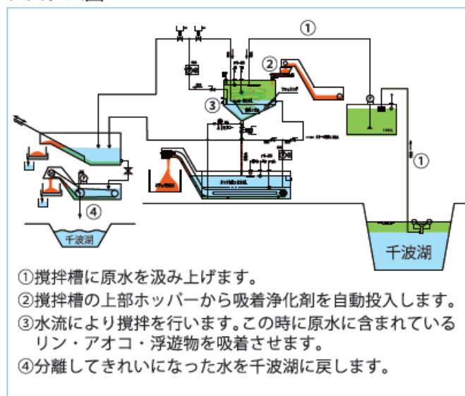
システム図
